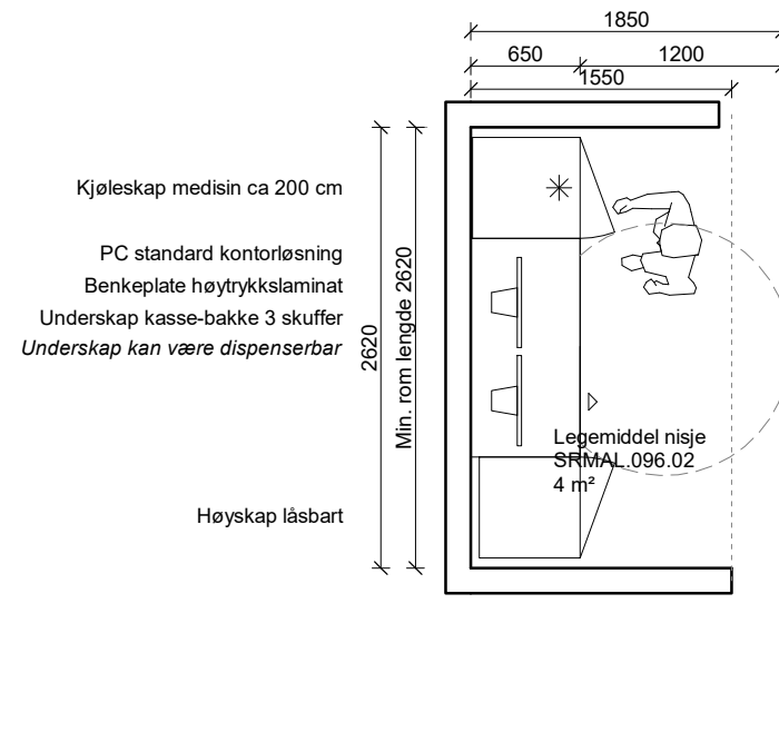
Legemiddel - Nisje | 1 : 50
